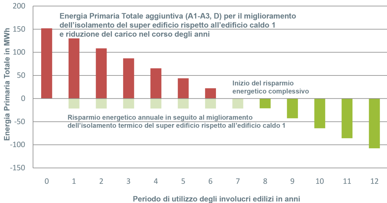
Figura 25: Ammortamento dell'incremento di isolamento termico grazie al risparmio energetico lungo il periodo di utilizzo
