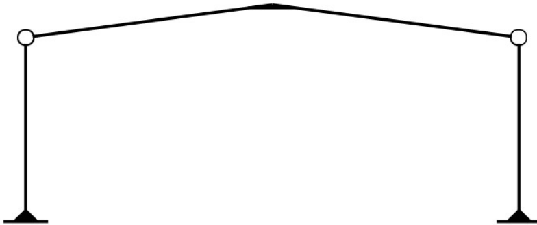
Figura 5: Schema statico di trave incernierata a pilastri incastrati alla base
