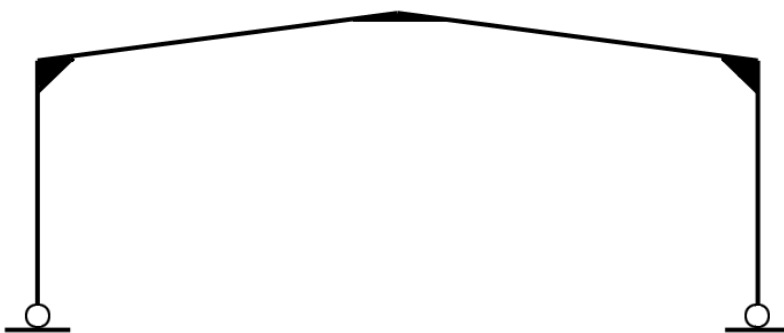
Figura 3: Schema statico di telaio a portale incernierato alla base
