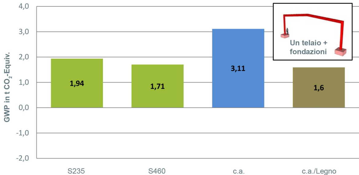
Figura 11: Potenziale di riscaldamento globale per la fase di prodotto (A1-A3) sommato ai costi & benefici (D) da riciclo (acciaio), incenerimento (legno) o trattamento delle macerie (calcestruzzo) per un telaio con fondazioni, in t di CO 2 equivalenti
