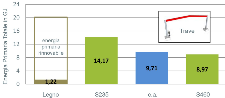
Figura 21: Energia primaria totale per la fase di prodotto (A1-A3) sommata ai costi & benefici (D) da riciclo (acciaio), incenerimento (legno) o trattamento delle macerie (calcestruzzo) per una trave, in GJ
