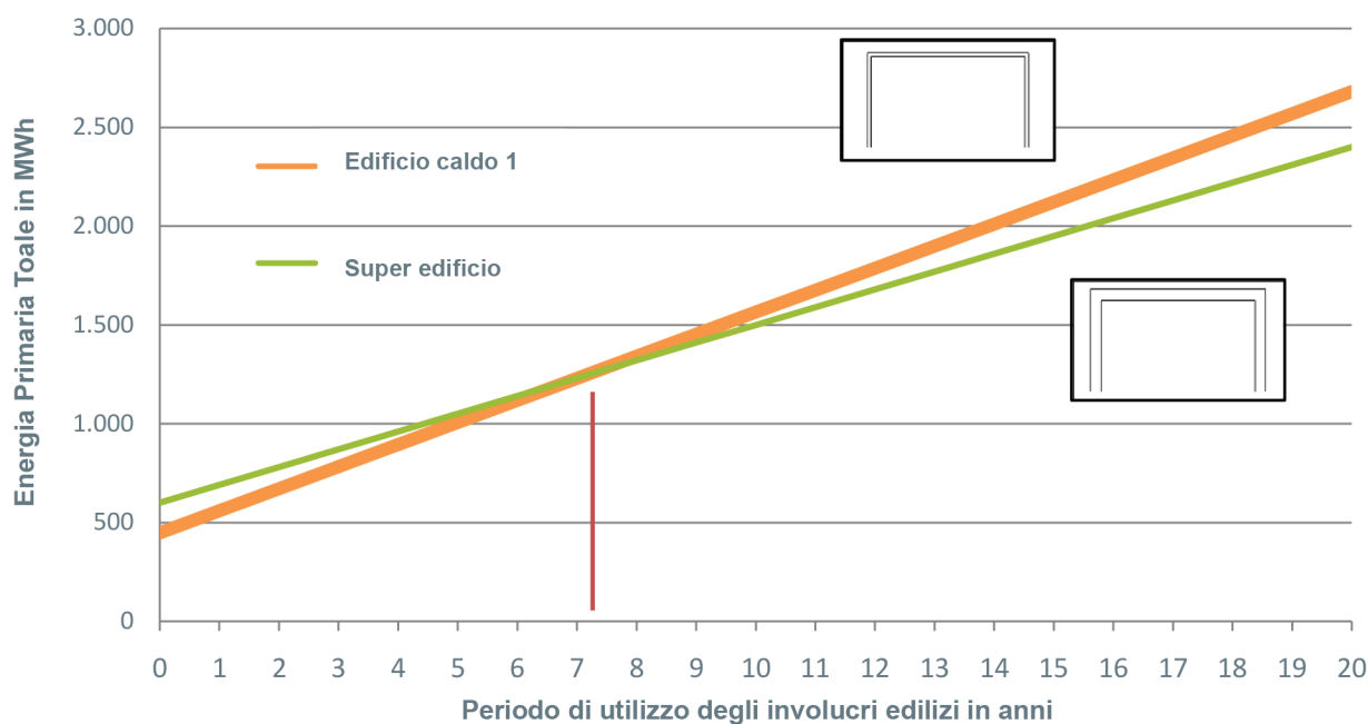
Figura 24: Confronto del consumo di energia primaria per l'involucro edilizio dell'edificio caldo 1 e del super edificio lungo un periodo di utilizzo di 20 anni, inclusi la fase di prodotto (A1-A3), costi & benefici (D) e il consumo energetico in esercizio (B6)
