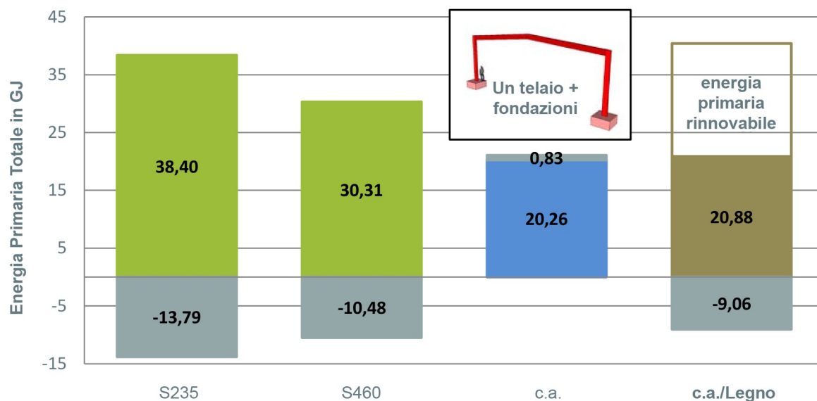
Figura 12: Energia primaria totale per la fase di prodotto (A1-A3) e separatamente costi & benefici (D, grigio) da riciclo (acciaio), incenerimento (legno) o trattamento delle macerie (calcestruzzo) per un telaio con fondazioni, in GJ
