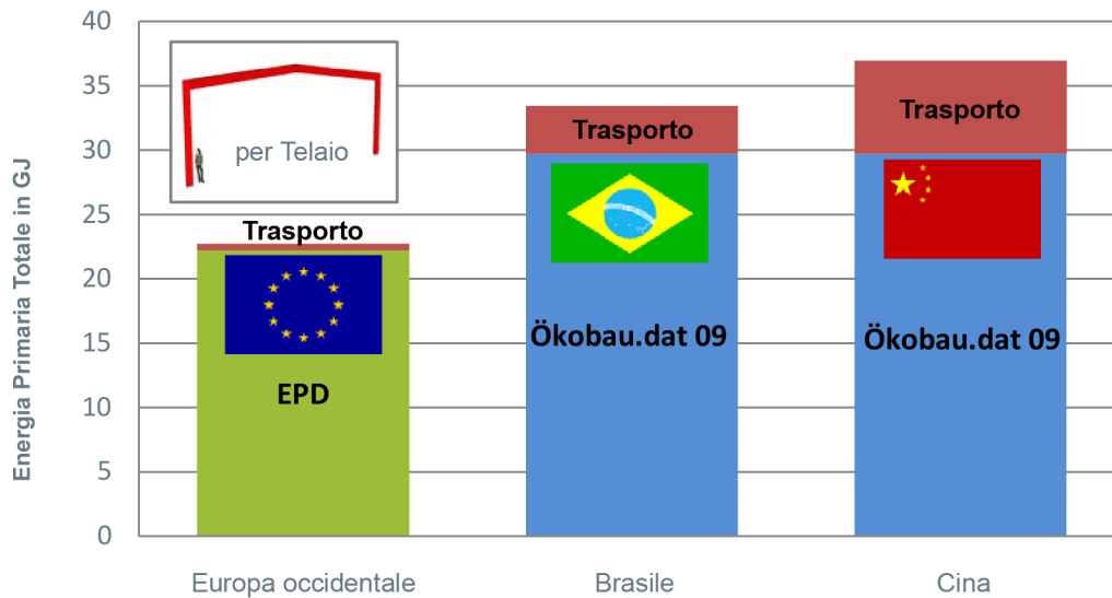
Figura 27: Energia primaria totale per un telaio in acciaio S235 incluso il trasporto (A4) dal “cancello” al sito, in GJ
