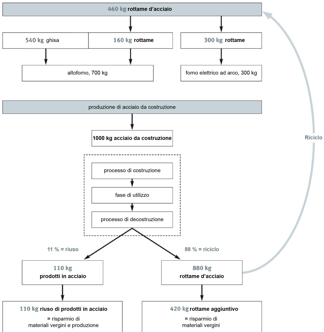
Figura 8: Individuazione schematica del Potenziale di Riciclo (rottame netto e prodotti in acciaio riutilizzati che rimpiazzano nuova produzione da minerale di ferro)
