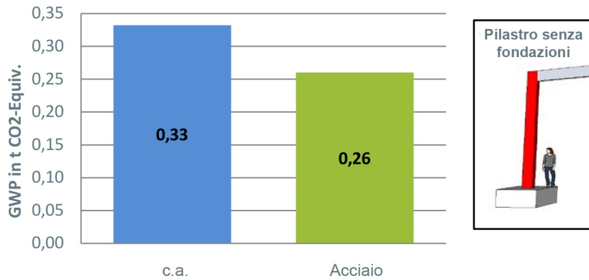
Figura 17: Potenziale di riscaldamento globale per la fase di prodotto (A1-A3) sommato ai costi & benefici (D) da riciclo (acciaio), incenerimento (legno) o trattamento delle macerie (calcestruzzo) per un pilastro senza fondazioni, in t di CO2 equivalenti
