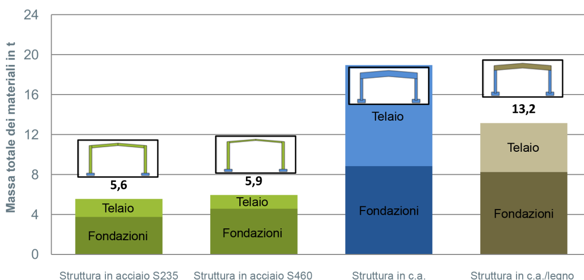
Figura 9: Quantità impiegate per i diversi sistemi costruttivi: telai e fondazioni, in t
