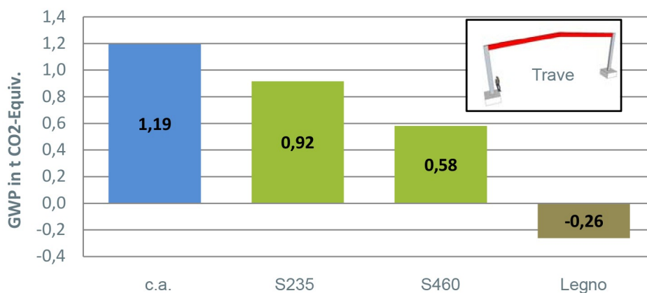
Figura 20: Potenziale di riscaldamento globale per la fase di prodotto (A1-A3) sommato ai costi & benefici (D) da riciclo (acciaio), incenerimento (legno) o trattamento delle macerie (calcestruzzo) per una trave, in t di CO2 equivalenti
