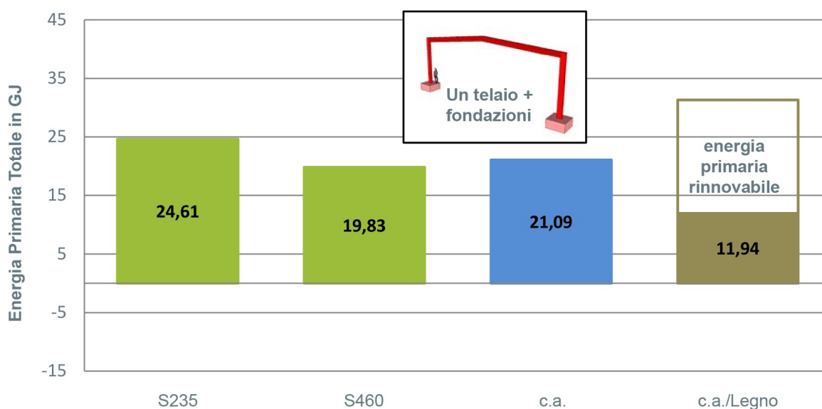
Figura 13: Energia primaria totale per la fase di prodotto (A1-A3) sommata ai costi & benefici (D) da riciclo (acciaio), incenerimento (legno) o trattamento delle macerie (calcestruzzo) per un telaio con fondazioni, in GJ
