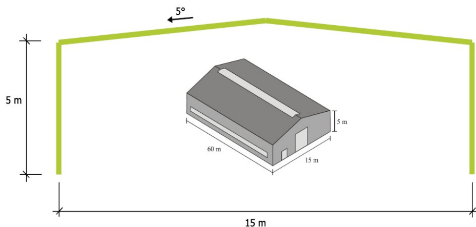
Figura 2: Dimensioni dell'edificio a singola elevazione e del relativo telaio strutturale
