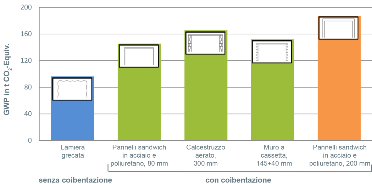
Figura 22: Potenziale di riscaldamento globale per la fase di prodotto (A1-A3) sommato ai costi & benefici (D) per le pareti esterne, in t di CO 2 equivalenti
