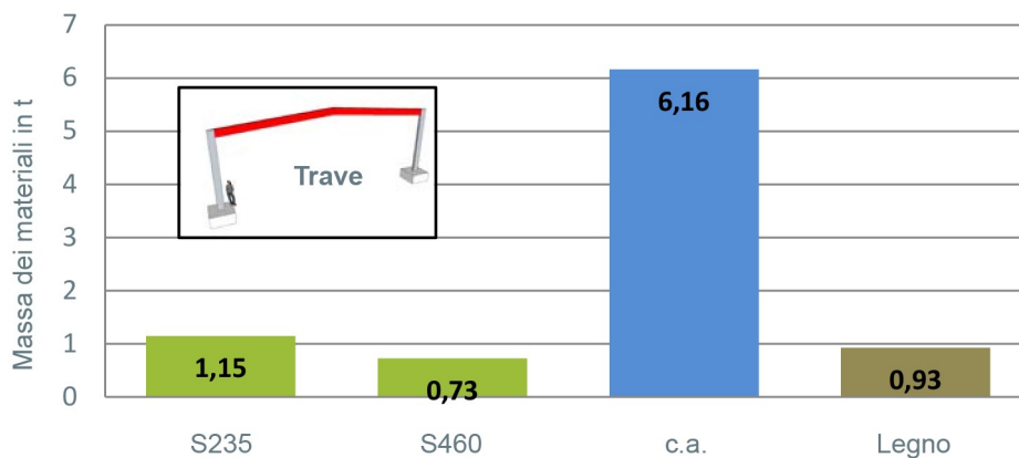
Figura 19: Quantità per una trave, in t
