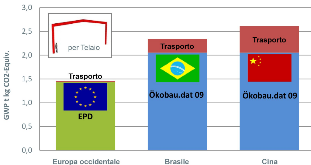
Figura 26: Potenziale di riscaldamento globale per un telaio in acciaio S235 incluso il trasporto (A4) dal “cancello” al sito, in CO 2 equivalenti
