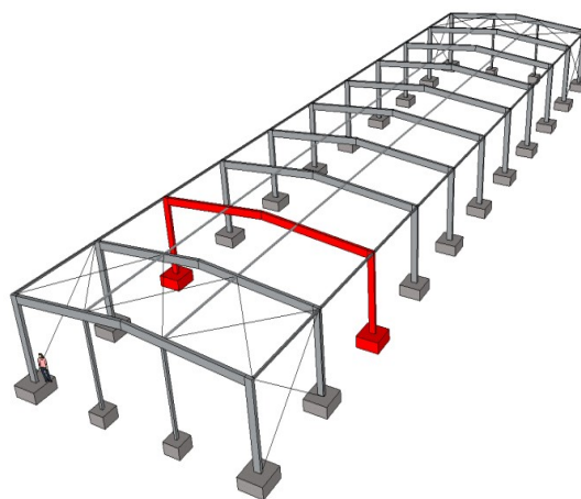
Figura 1: Vista prospettica del sistema strutturale di un edificio a singola elevazione, con la struttura base intelaiata, vista come unità funzionale
