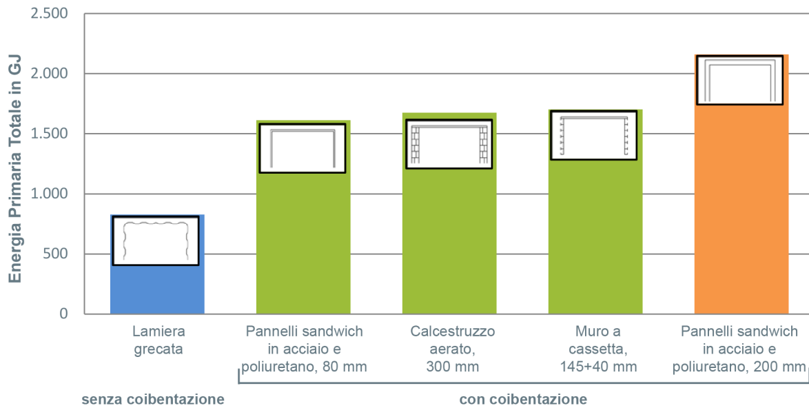
Figura 23: Energia primaria totale per la fase di prodotto (A1-A3) sommata ai costi & benefici (D) per le pareti esterne, in t di CO 2 equivalenti
