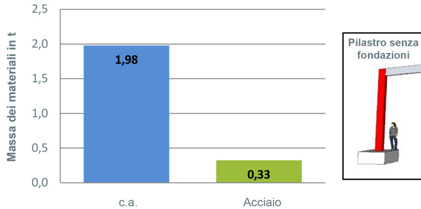
Figura 16: Quantità per pilastri senza fondazioni, in t
