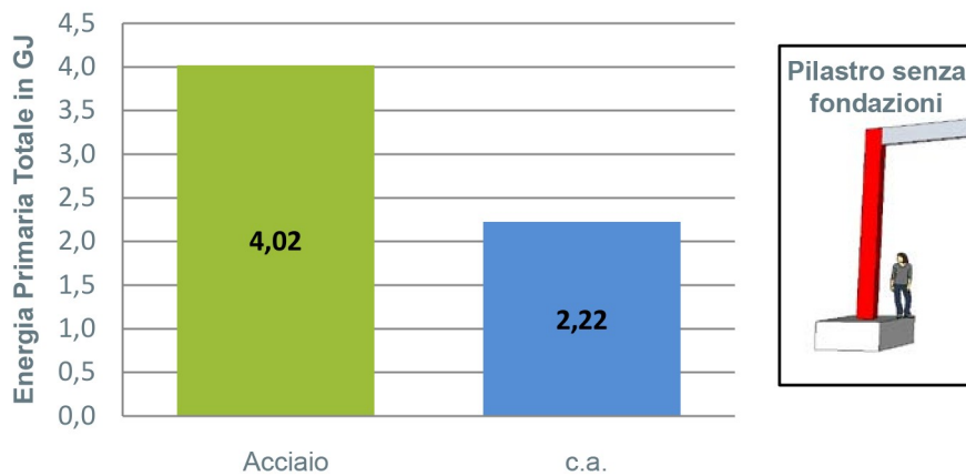
Figura 18: Energia primaria totale per la fase di prodotto (A1-A3) sommato ai costi & benefici (D) da riciclo (acciaio), incenerimento (legno) o trattamento delle macerie (calcestruzzo) per un pilastro senza fondazioni, in GJ
