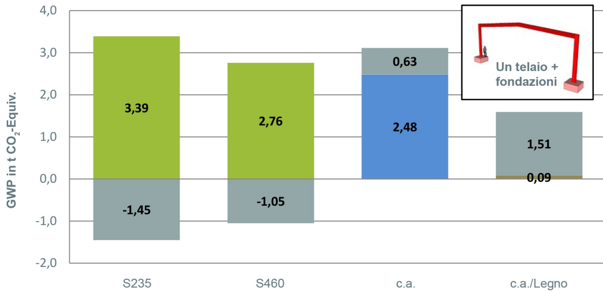
Figura 10: Potenziale di riscaldamento globale per la fase di prodotto (A1-A3) e separatamente costi & benefici (D, grigio) da riciclo (acciaio), incenerimento (legno) o trattamento delle macerie (calcestruzzo) per un telaio con fondazioni, in t di CO 2 equivalenti
