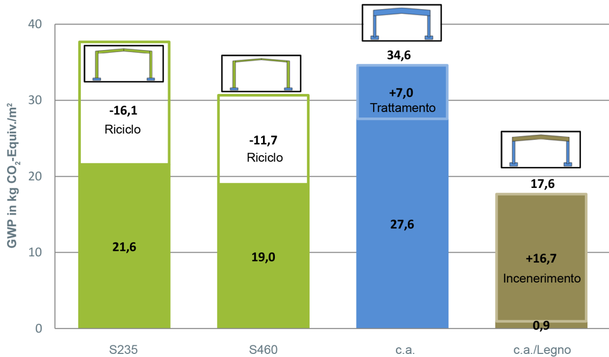
Figura 14: Potenziale di riscaldamento globale per la fase di prodotto (AI-A3) sommato ai costi & benefici (D) da riciclo (acciaio), incenerimento (legno) o trattamento delle macerie (calcestruzzo) per un telaio con fondazioni, in kg di CO 2 equivalenti per m 2 di superficie calpestabile
