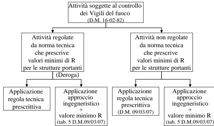
Figura 1 - Procedure per determinare i requisiti minimi di resistenza al fuoco delle strutture portanti di una costruzione.
